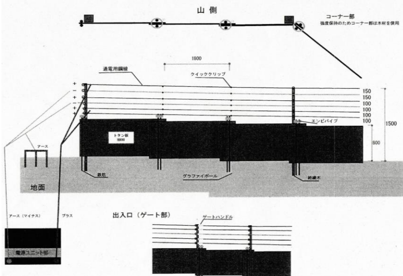
電気柵の構造図
